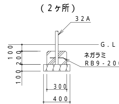
C基礎詳細図 S = 1 / 30
