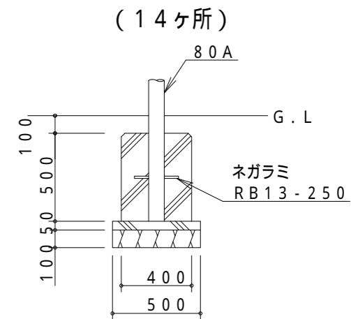
B基礎詳細図 S = 1 / 30
