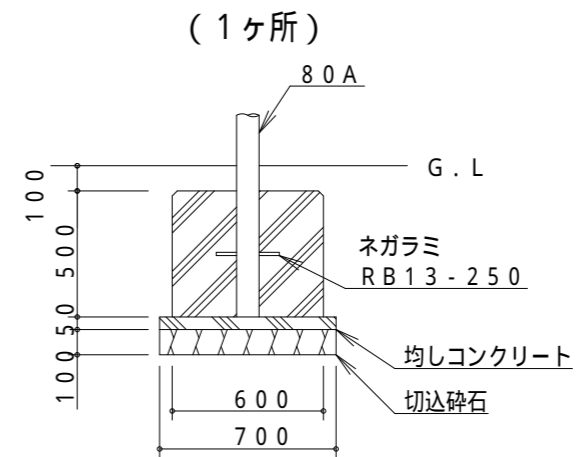
A基礎詳細図 S = 1 / 30
