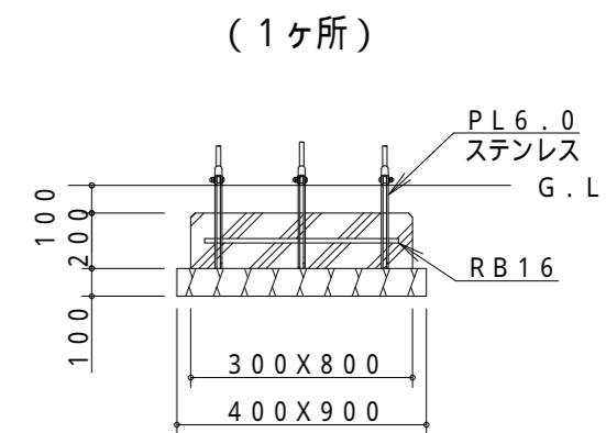
D基礎詳細図 S = 1 / 30
