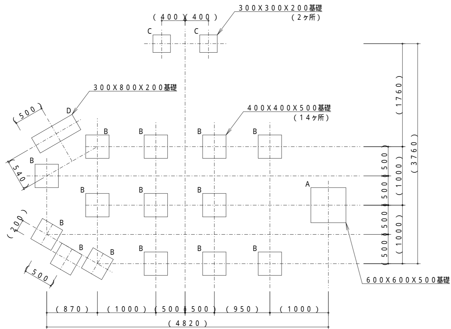
基礎平面図
