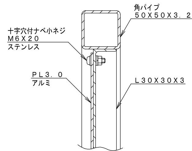
A-A断面図 S=1/3
