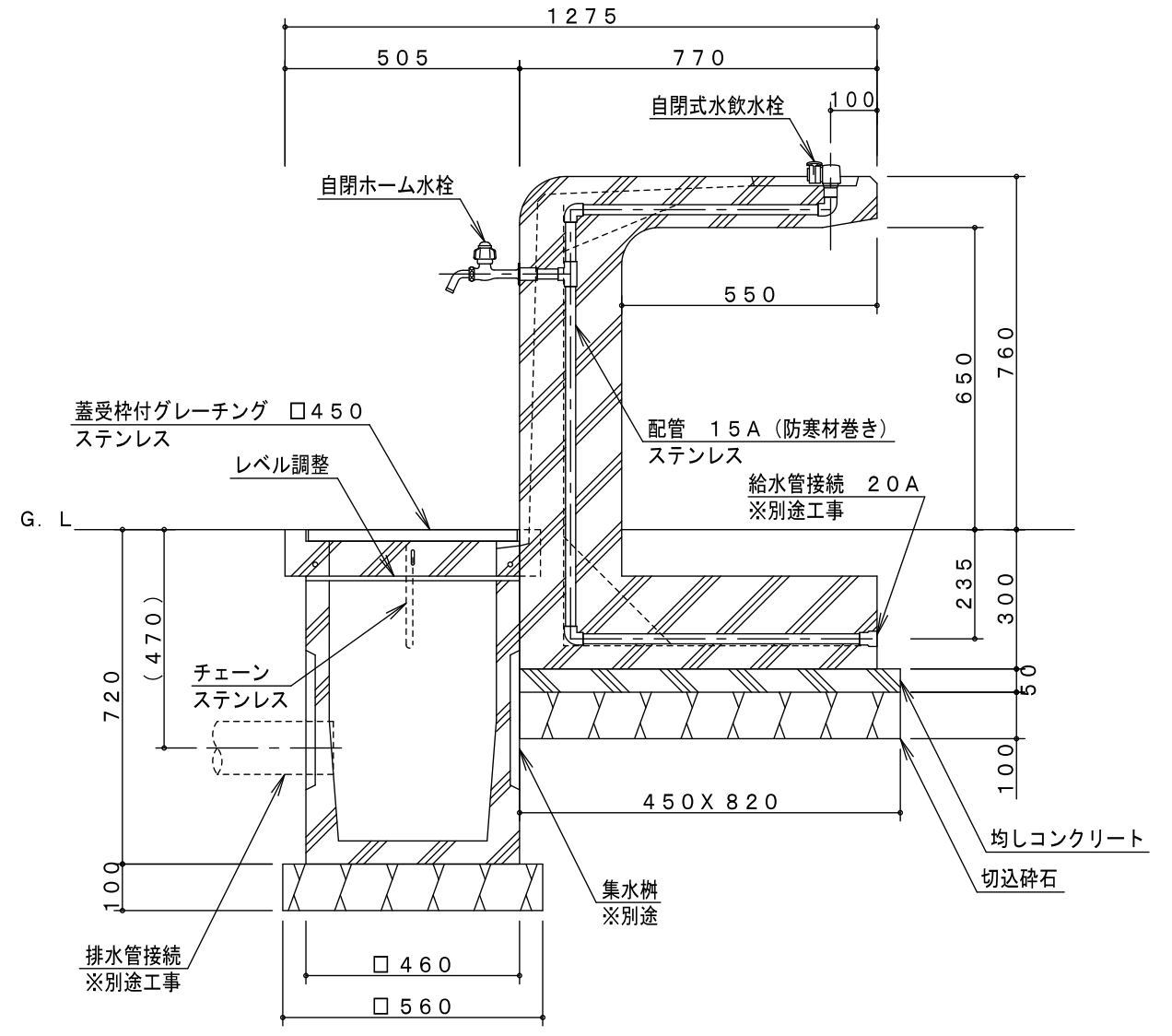
断面詳細図 S=1/15
